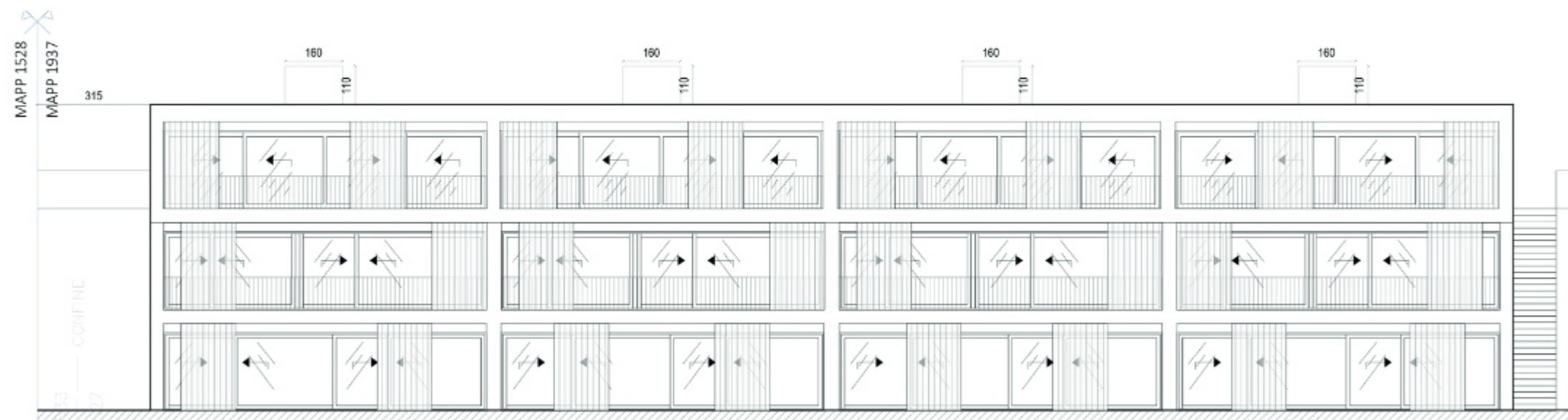
PROSPETTO SUD
